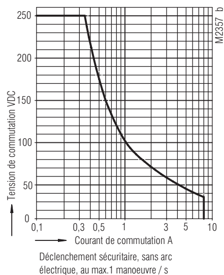
Courbe limite d'arc (contacts temporisé)
