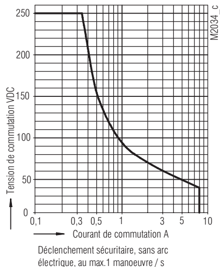
Courbe limite d'arc (contacts instantané)
